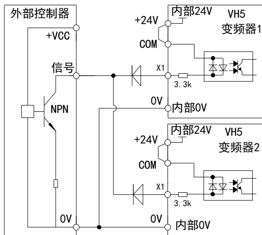
多台变频器使用变频器内24V电源的漏型接线方法
