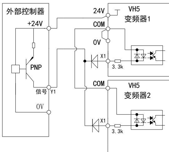
多台变频器使用变频器24V电源的源型接线方法
