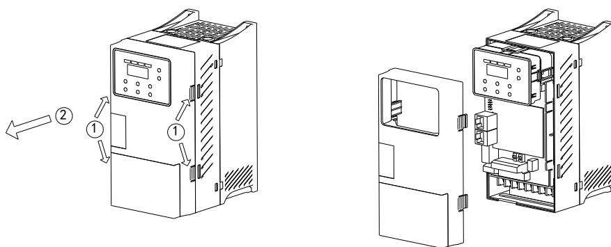
①双手按压上壳四处卡扣 ②沿箭头方向拿出来
