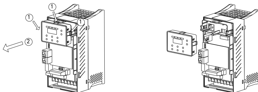
①用手按压控制器三处卡扣 ②沿箭头方向拿出来
